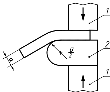
1 — тиски; 2 — оправка
